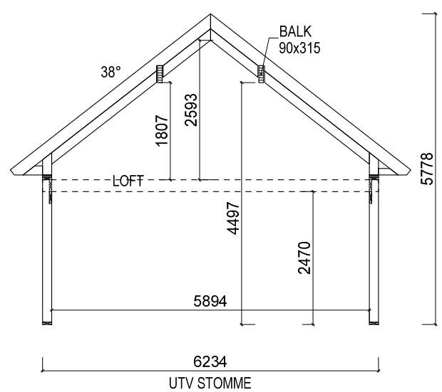
SEKTION A-A
