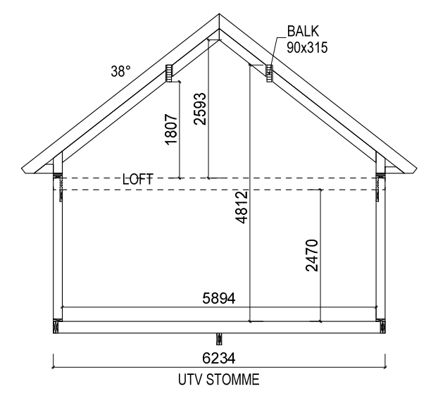
SEKTION A-A
