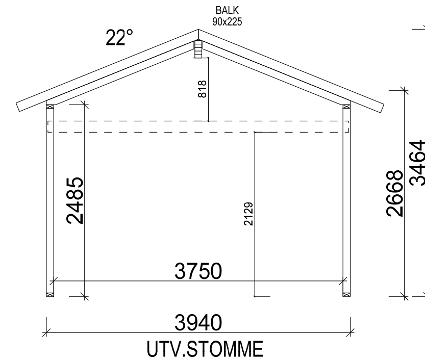
Sektion A-A
