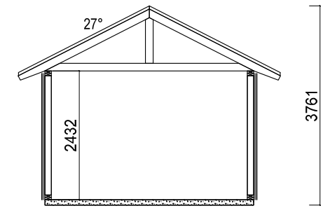
Sektion A-A
