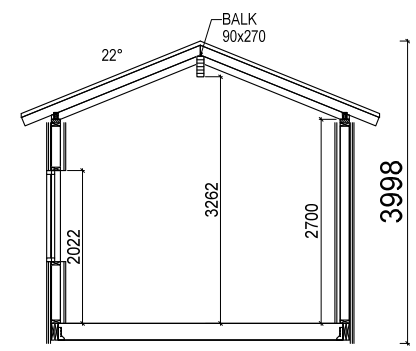
A-A
