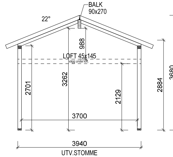
SEKTION A-A
