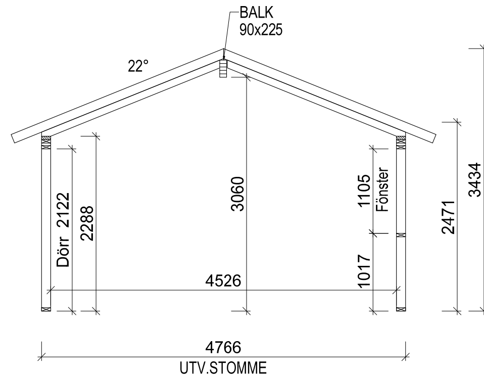
SEKTION A-A
