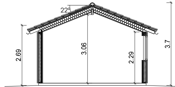
Sektion A-A
