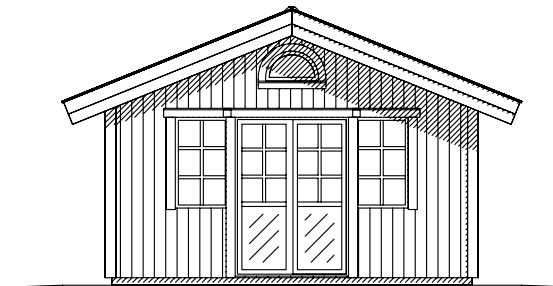
Fasad mot
