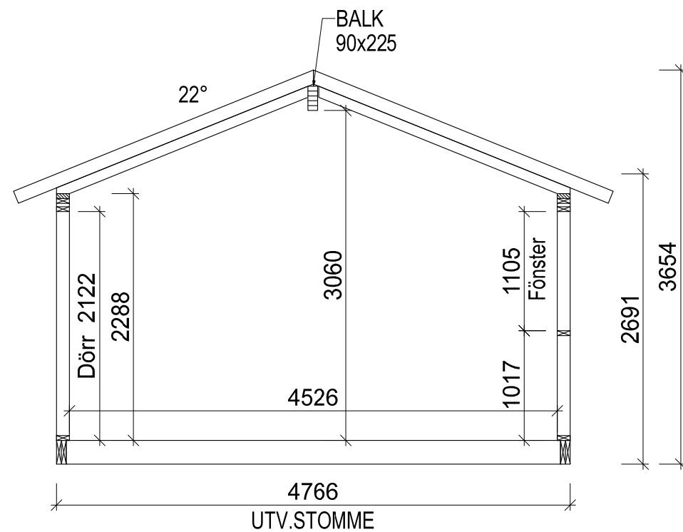
SEKTION A-A
