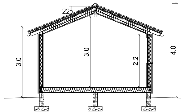
Sektion A-A
