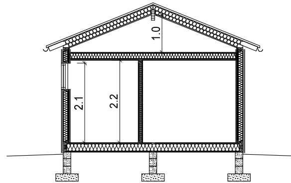
Sektion B-B
