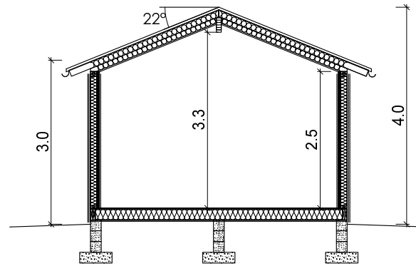
Sektion A-A
