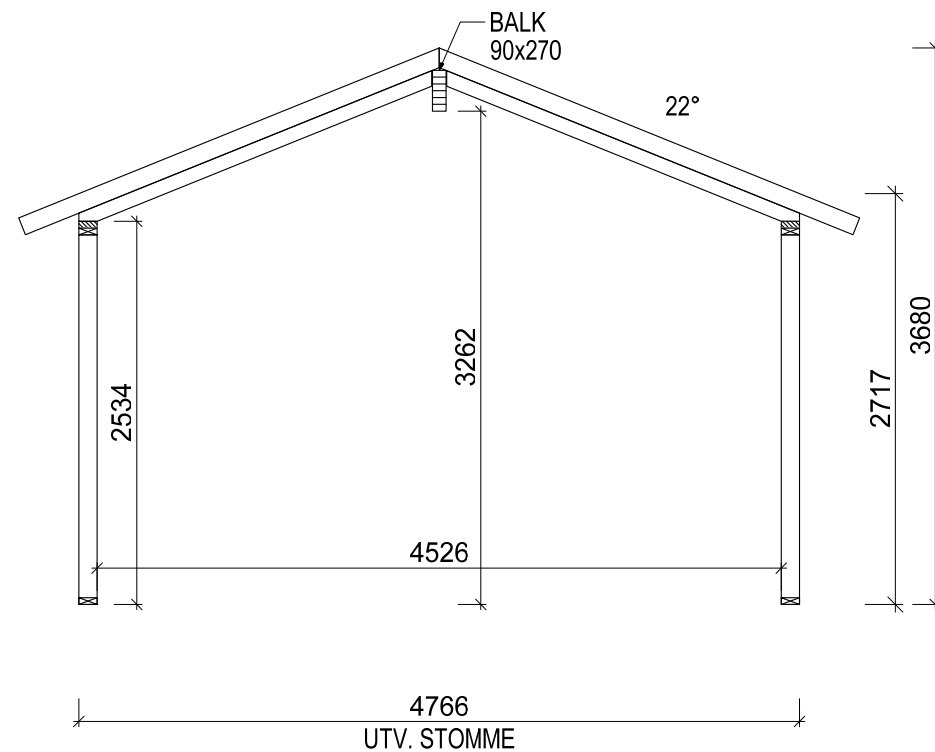
SEKTION A-A
