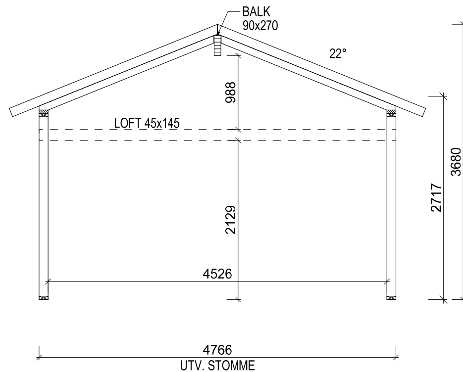
SEKTION B-B
