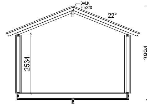
SEKTION A-A
