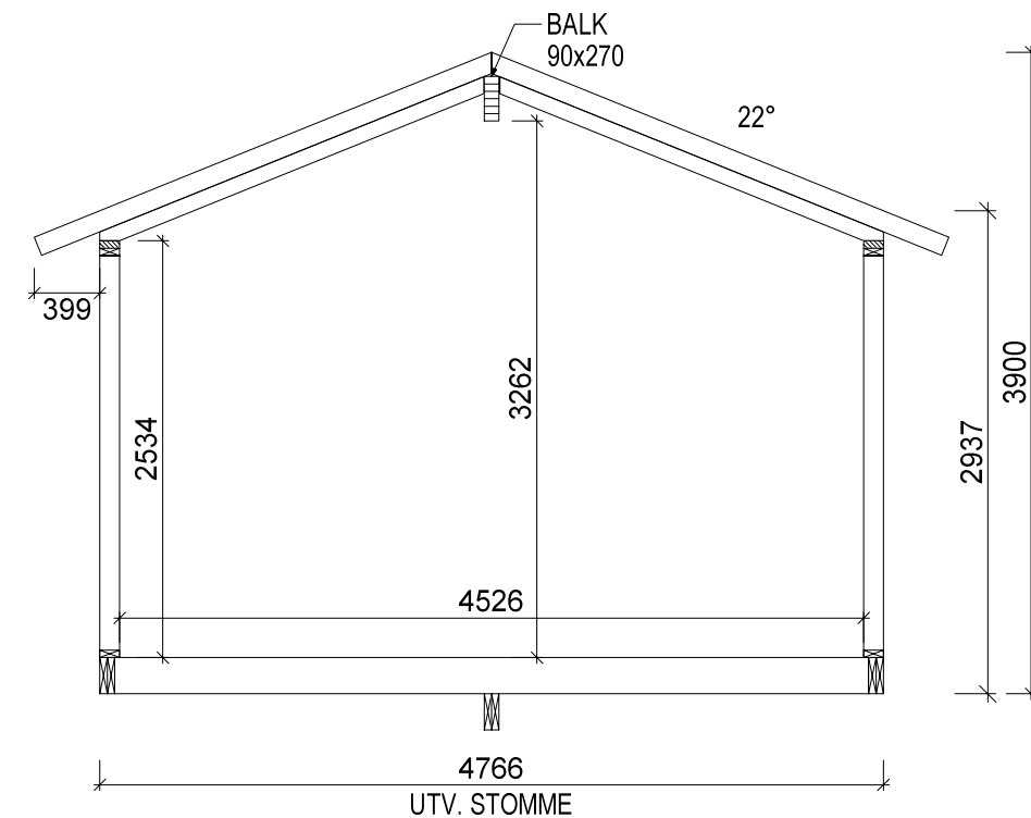
SEKTION A-A
