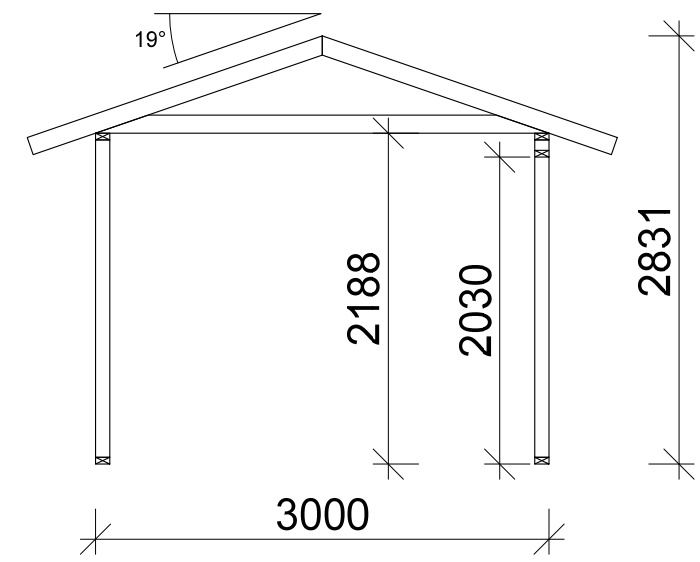
SEK A-A
