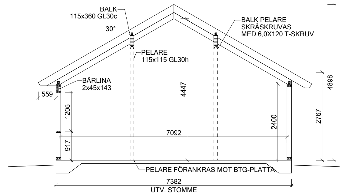
SEKTION A-A
