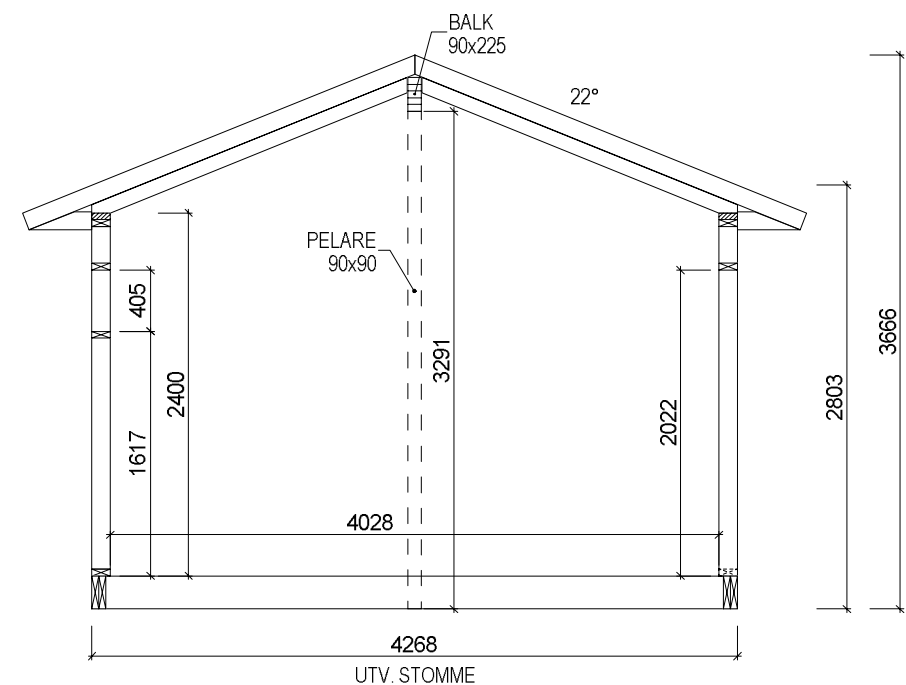
SEKTION A-A
