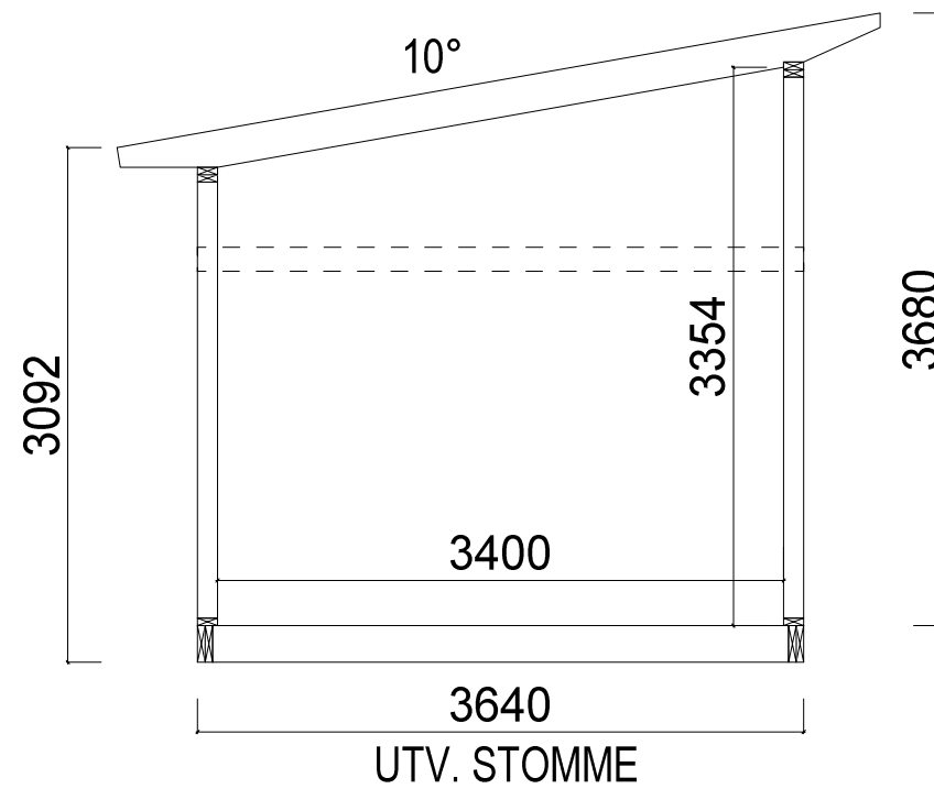
Sektion A-A
