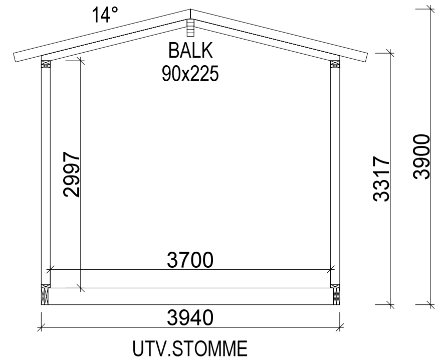
Sektion A-A
