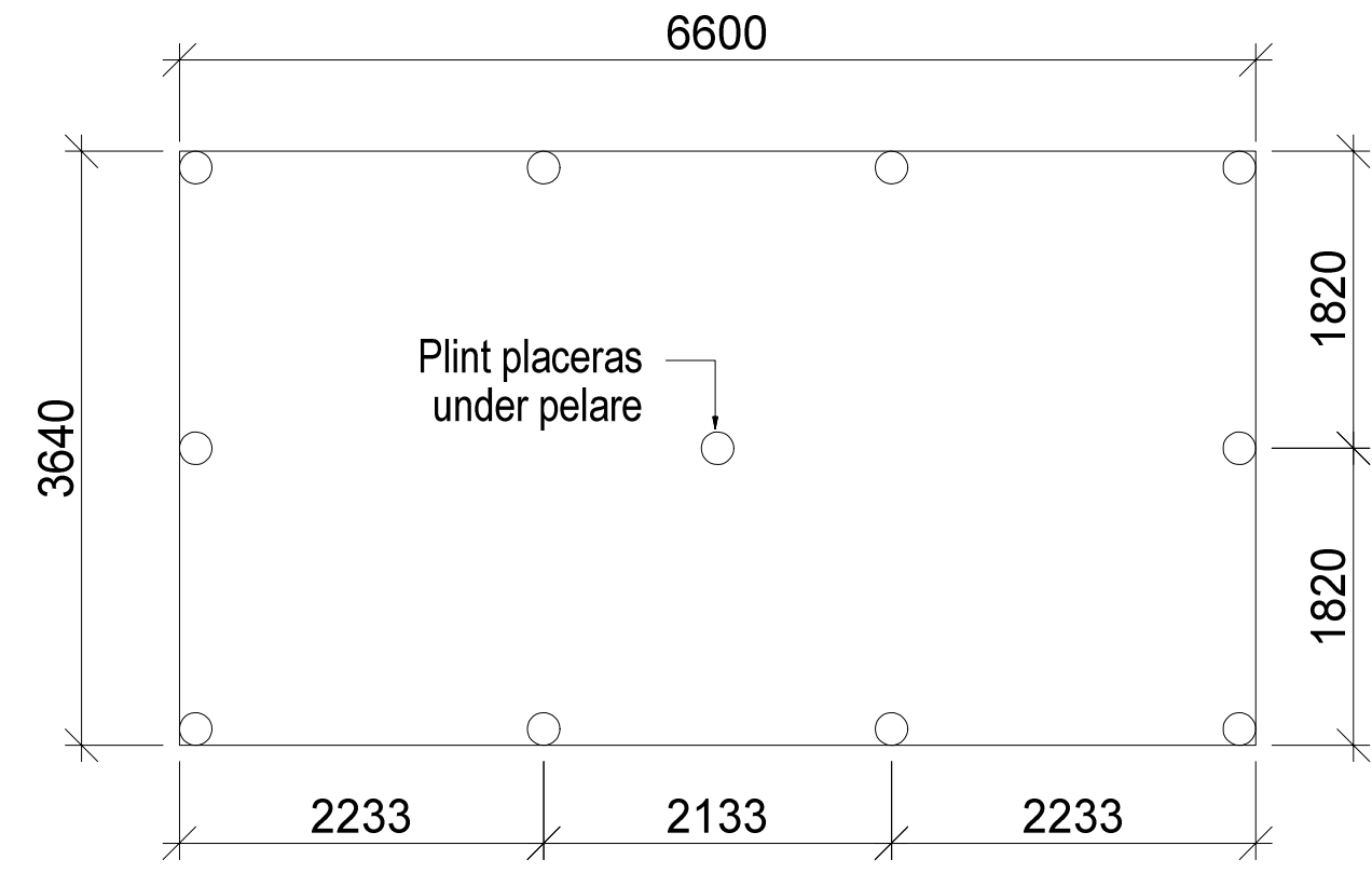
Plintgrund
