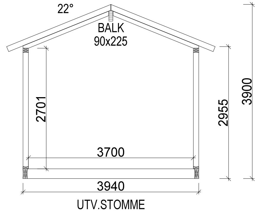
Sektion A-A
