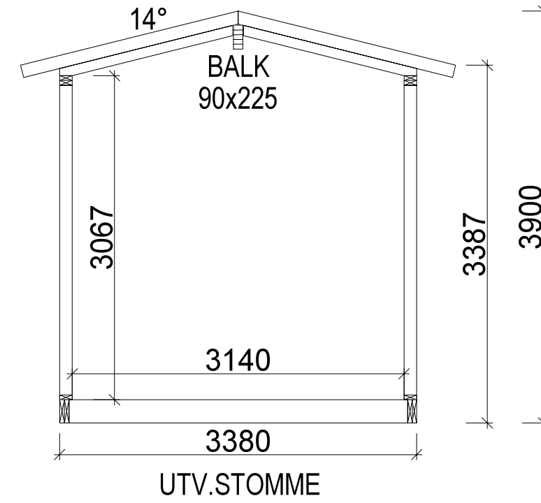
Sektion A-A
