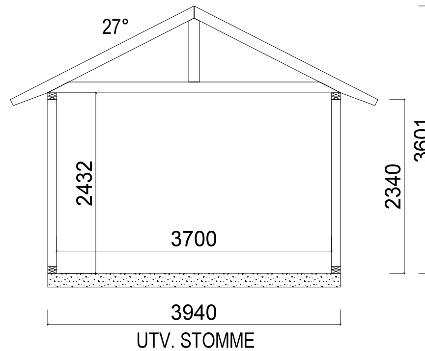
Sektion A-A
