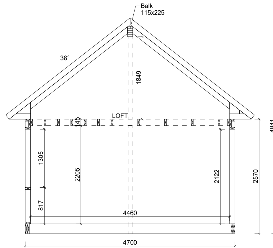
Sektion A-A
