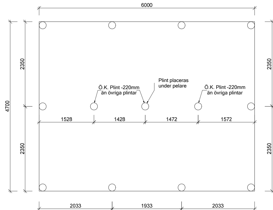
Plintgrund
