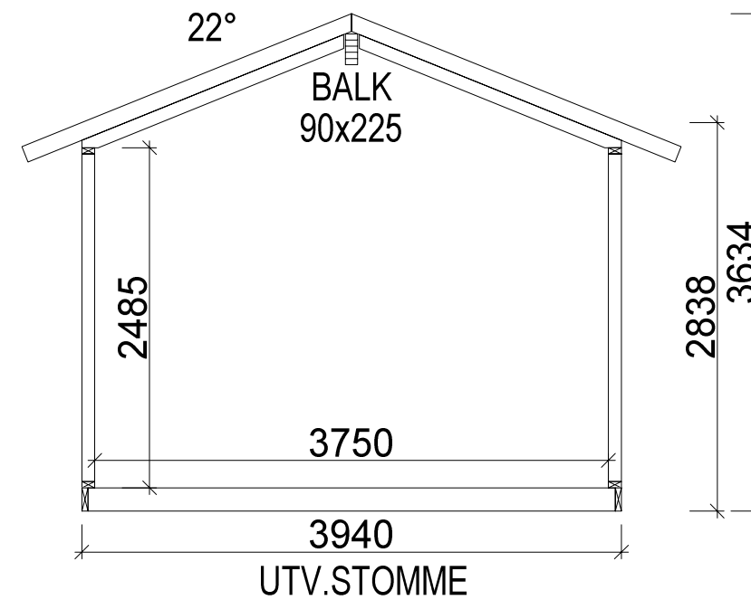
Sektion A-A
