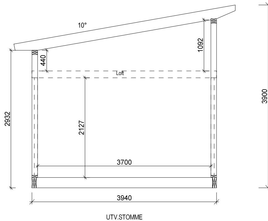
Sektion A-A
