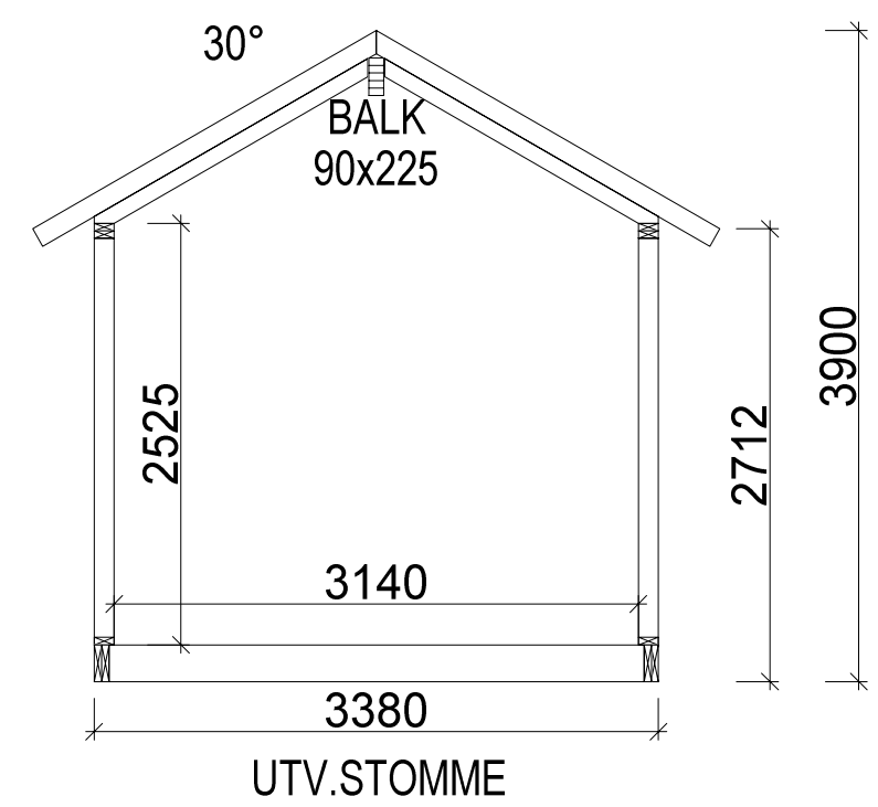
Sektion A-A
