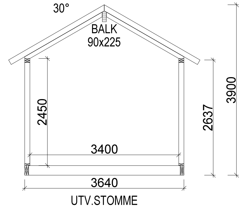
Sektion A-A
